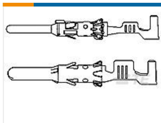
TE Part # 962972-7 2,5MM STIFTKONT EDS
